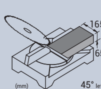
Corte 45°/90°: 65x165 mm
