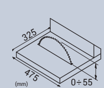
Corte con mesa: H. 55 mm
